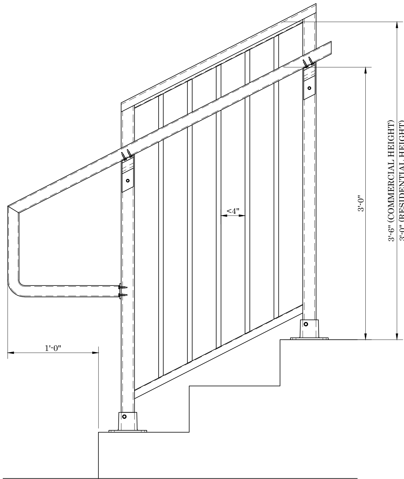
ELEVATION
