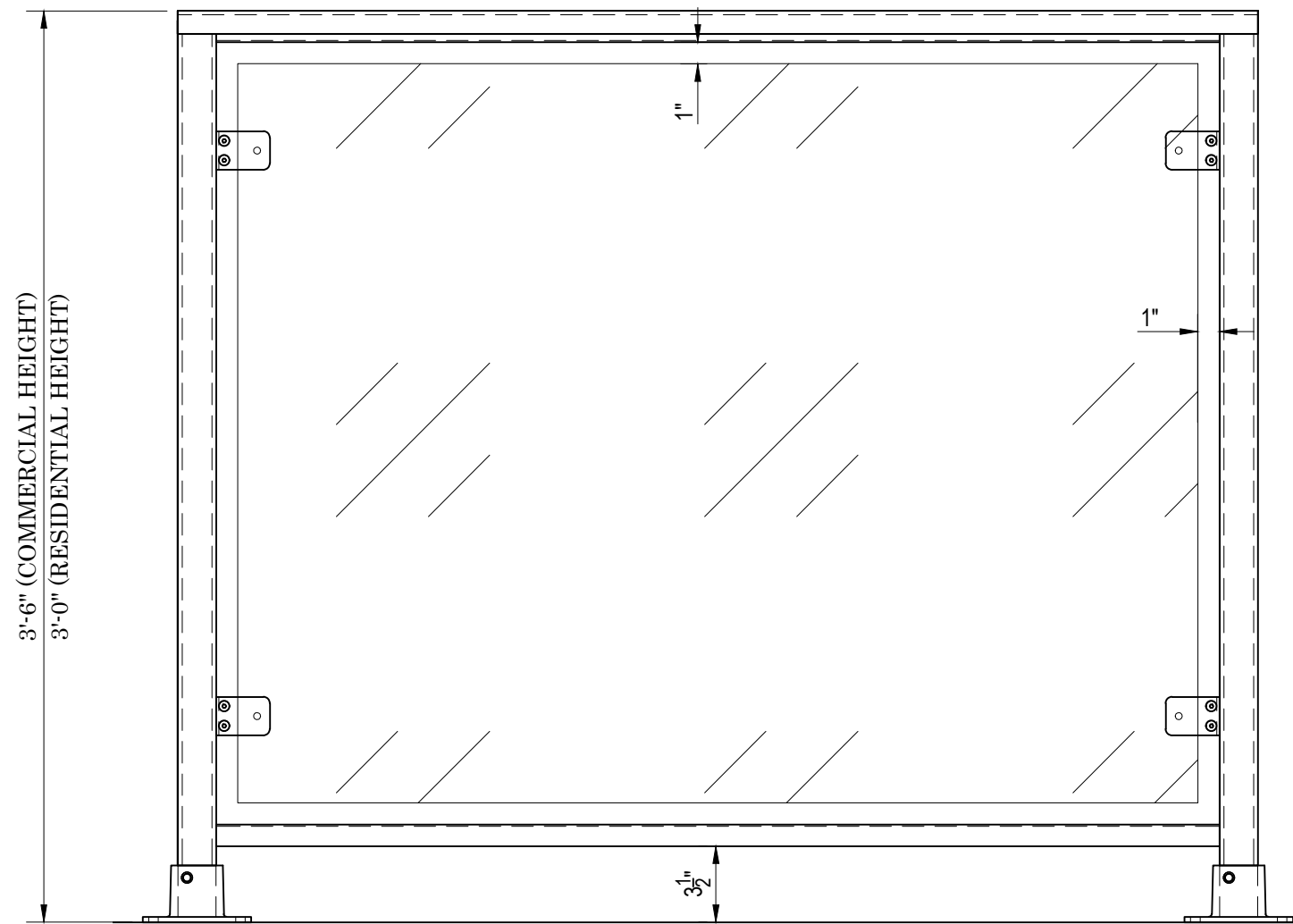
ELEVATION
